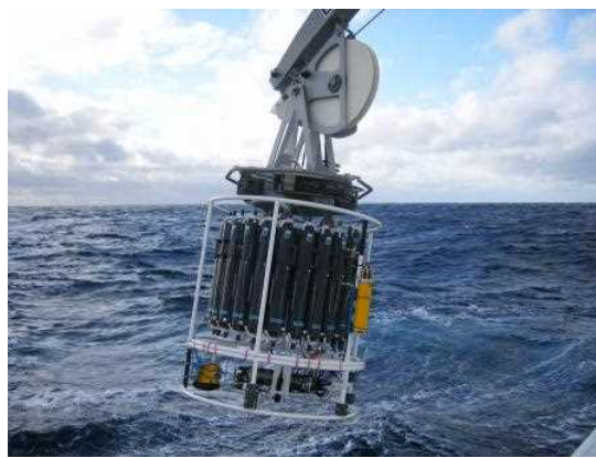
CTDによるモニタリング調査
